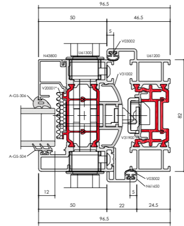
F82 LOCKING JAMB / C
